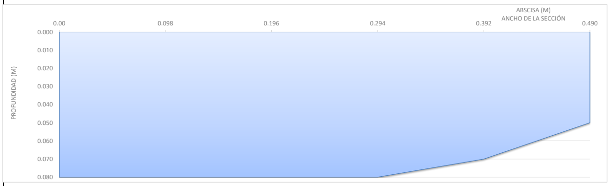
GRÁFICO ÁREA - SECCIÓN TRANSVERSAL DEL CAUCE
