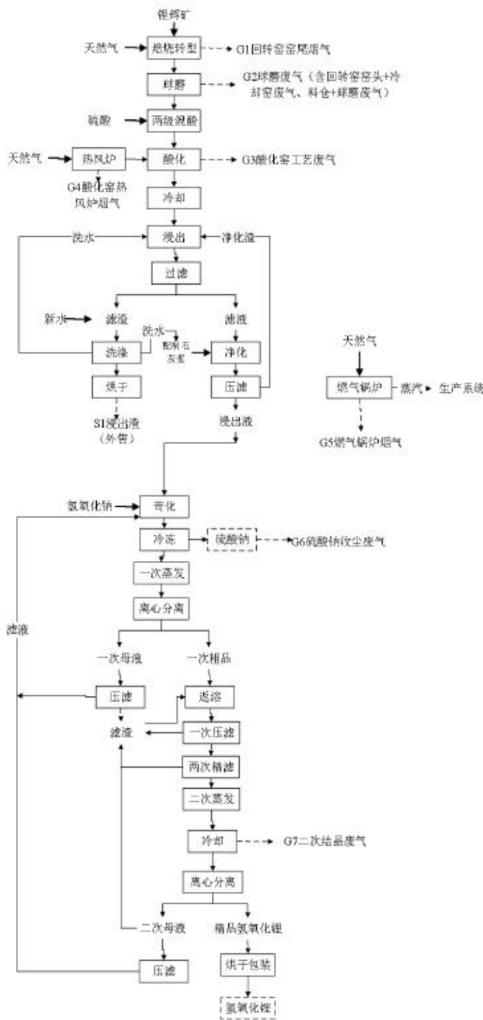
图 1 产品生产工艺流程图
